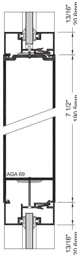
Traverse intermédiaire Mid rail 7 1/2" (190,5mm)
