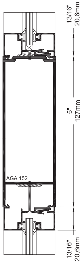
Traverse intermédiaire Mid rail 5" (127mm)
