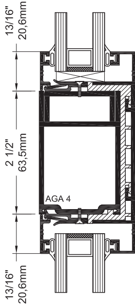
Traverse intermédiaire Mid rail 2 1/2" (63,5mm)
