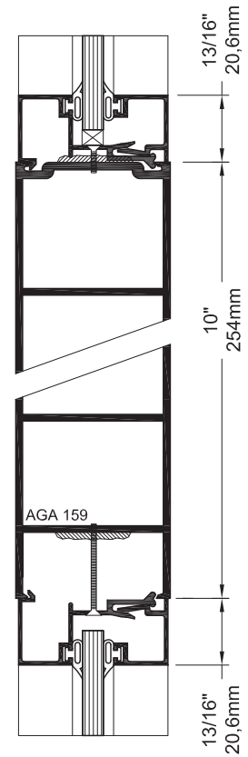
Traverse intermédiaire Mid rail 10" (254mm)
