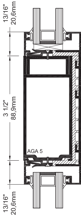
Traverse Intermédiaire Mid rail 3 1/2" (88,9mm)
