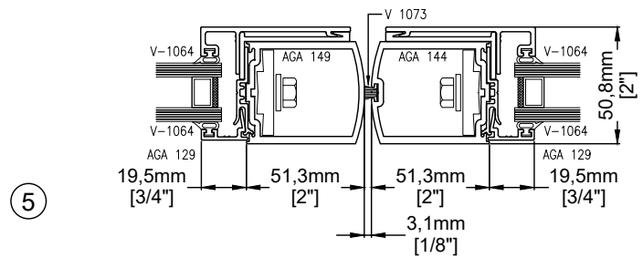
Charnière à mortaise continue Mortise continuous hinge
