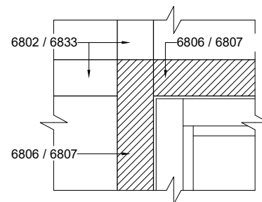
Élévation avec imposte Elevation with transom
