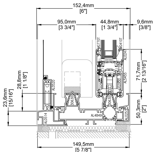
Panneau coulissant Sliding panel
