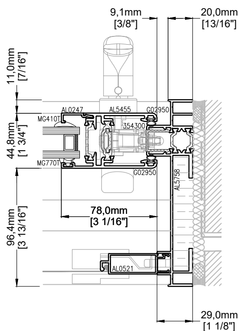
Panneau coulissant Sliding panel
